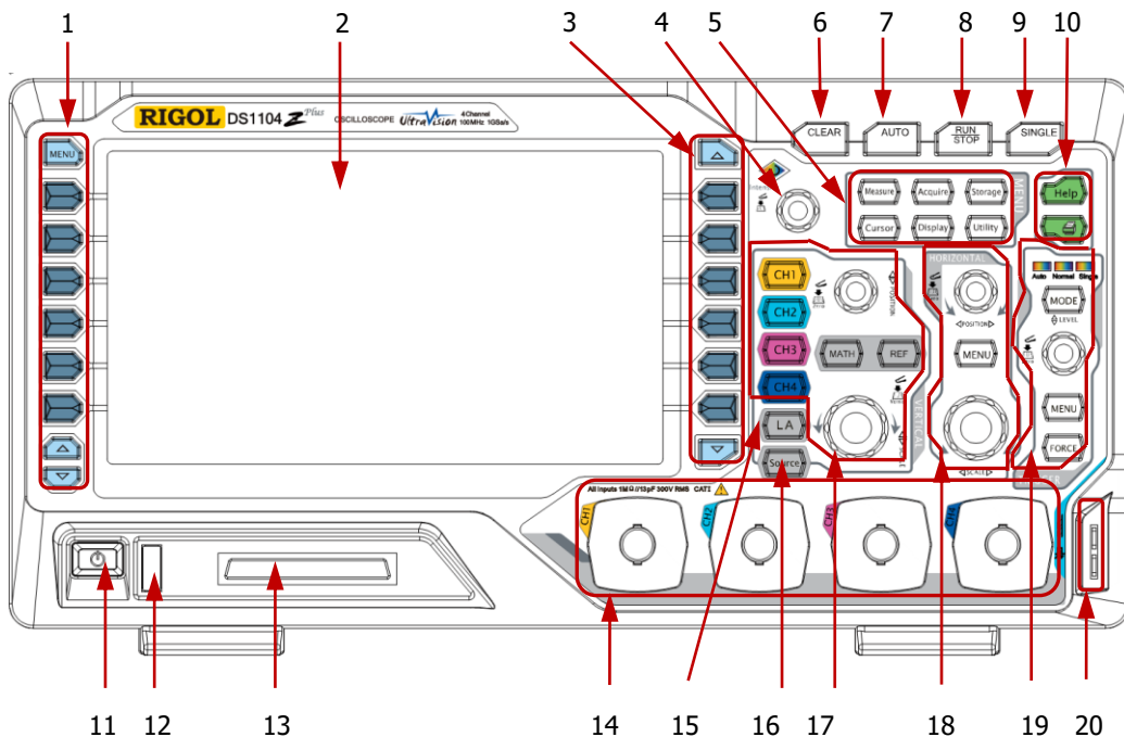
图 1-10 前面板总览
